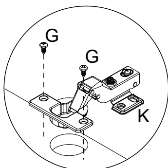
Detalhe 8 Detail/Detalle
