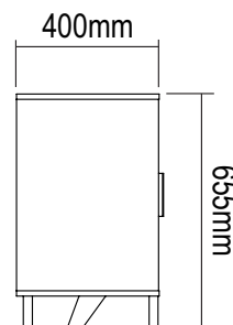
lateral/lado/side
