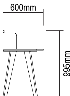
lateral/lado/side
