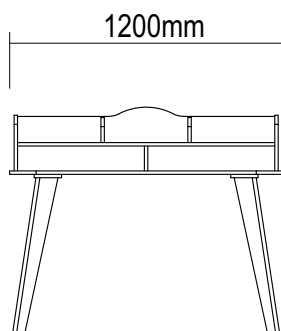
frente/frente/front
