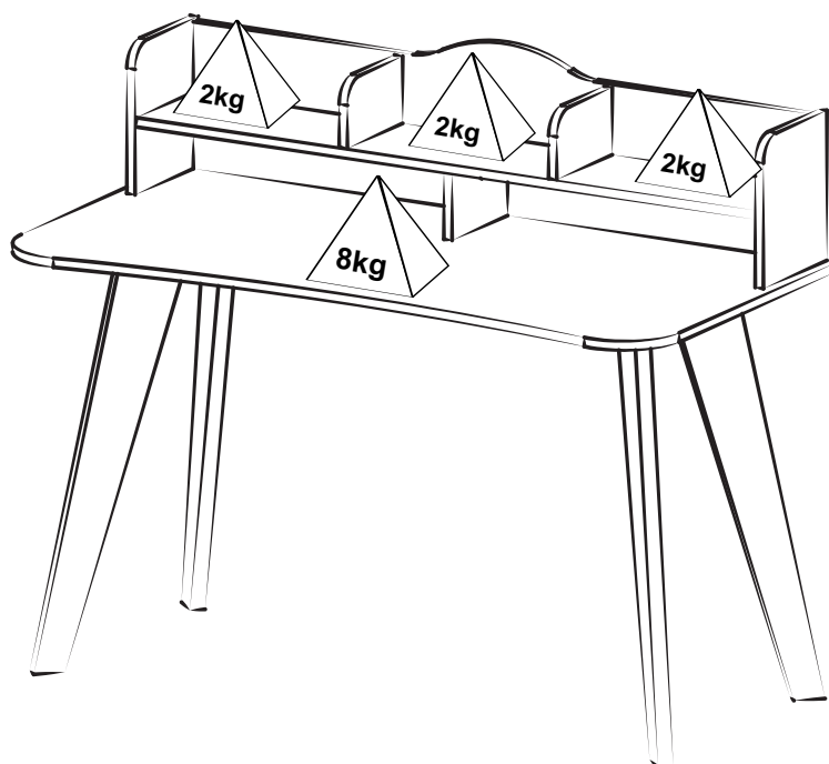
frente/frente/front
