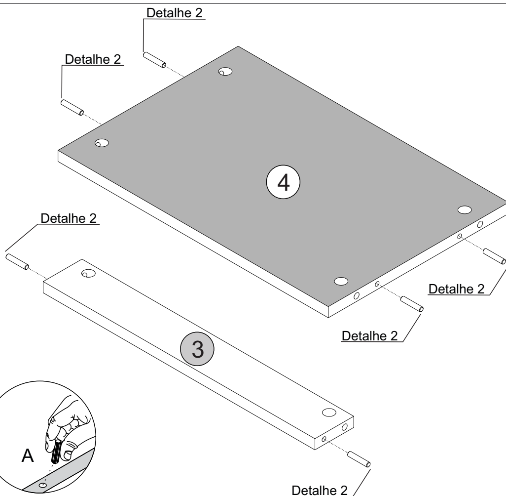
Detalhe 2 Detail/Detalle
