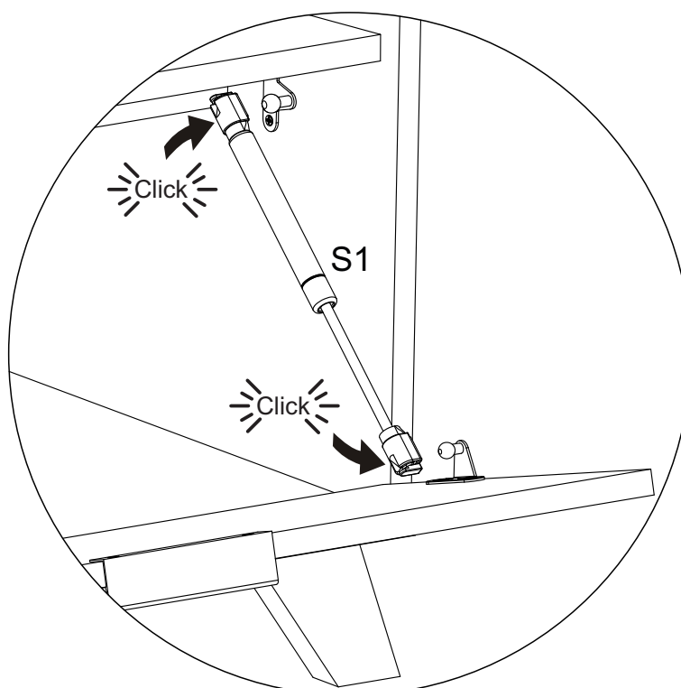
Detalhe 17
