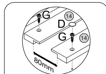
Detalhe 2 Detail/Detalle
