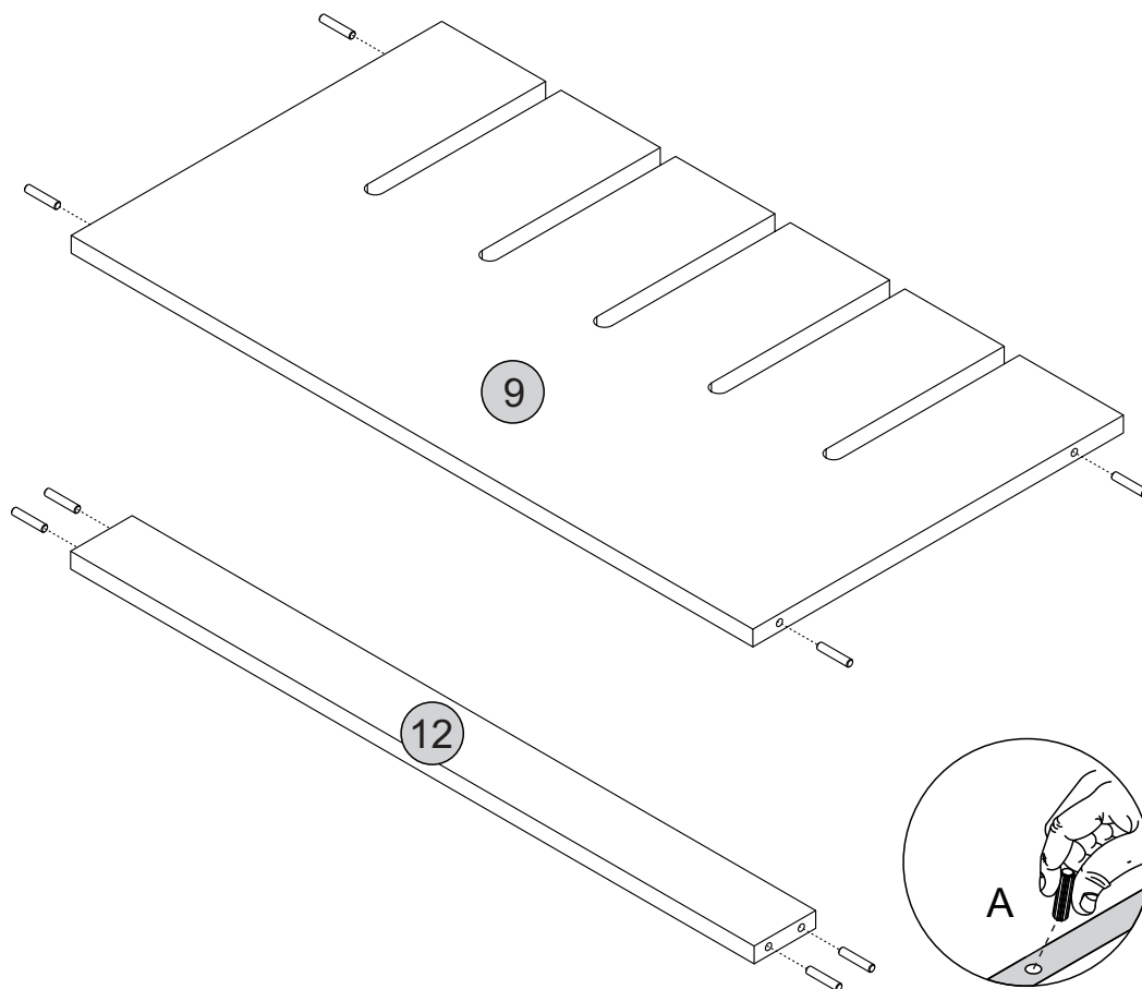
Detalhe 4 Detail/Detalle
