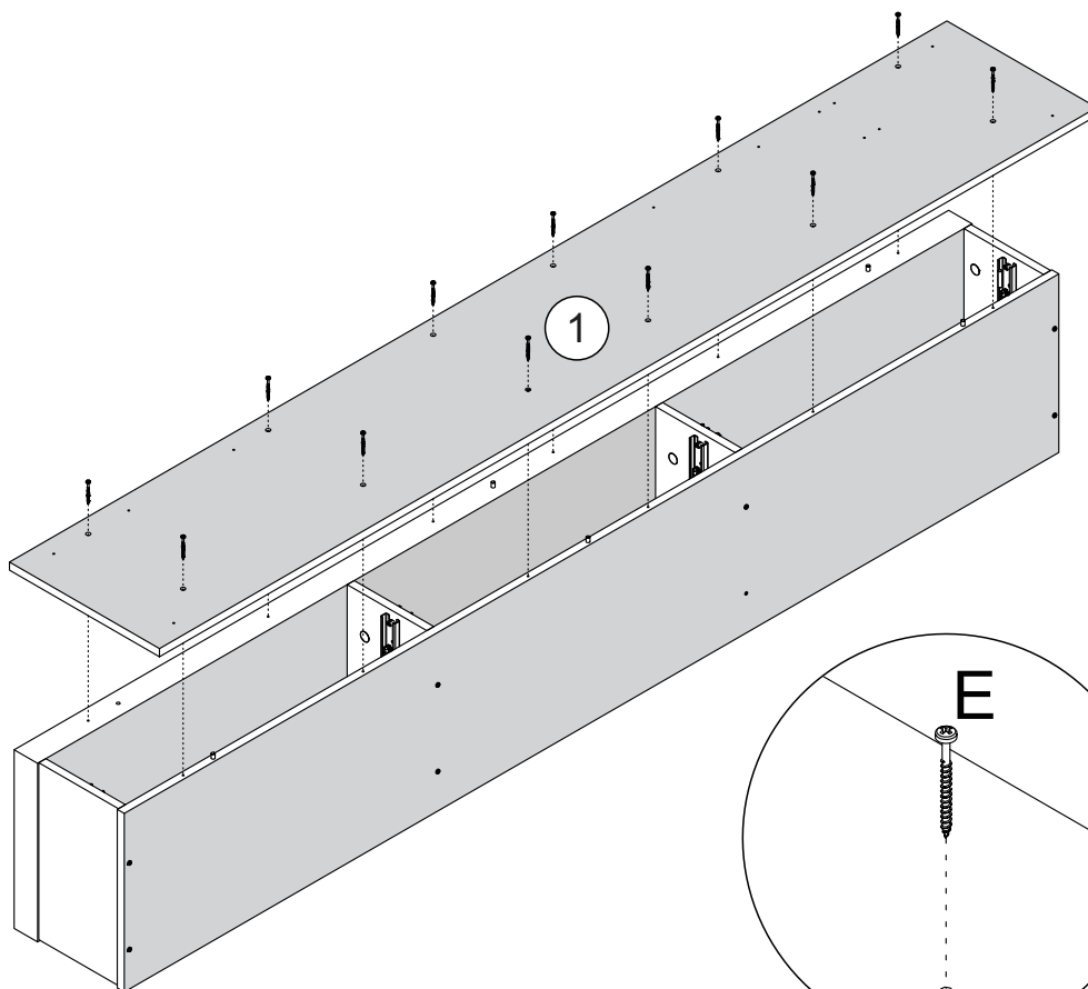
Detalhe 5 Detail/Detalle
