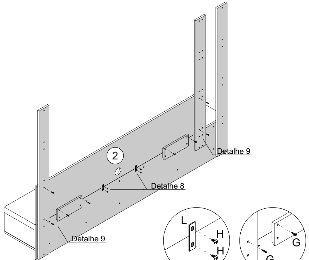
Detalhe 8 Detail/Detalle
