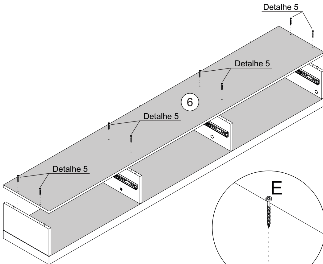
Detalhe 5 Detail/Detalle
