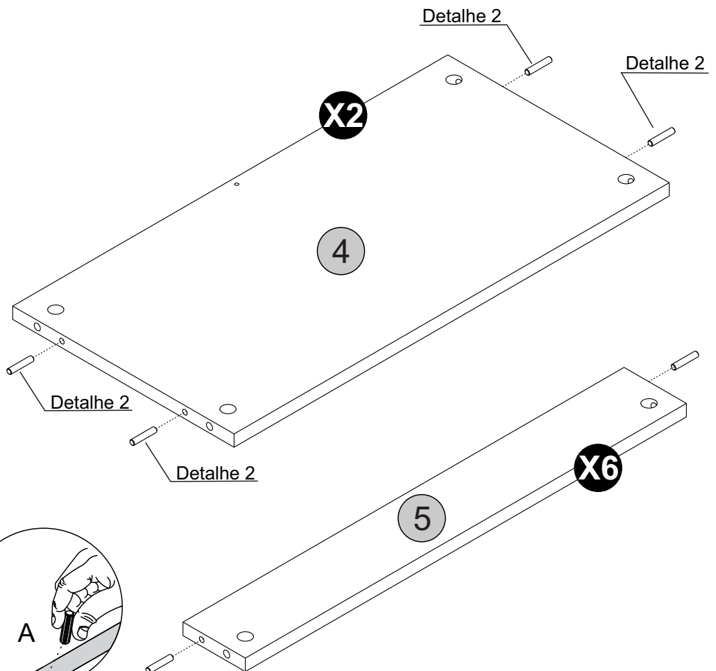
Detalhe 2 Detail/Detalle
