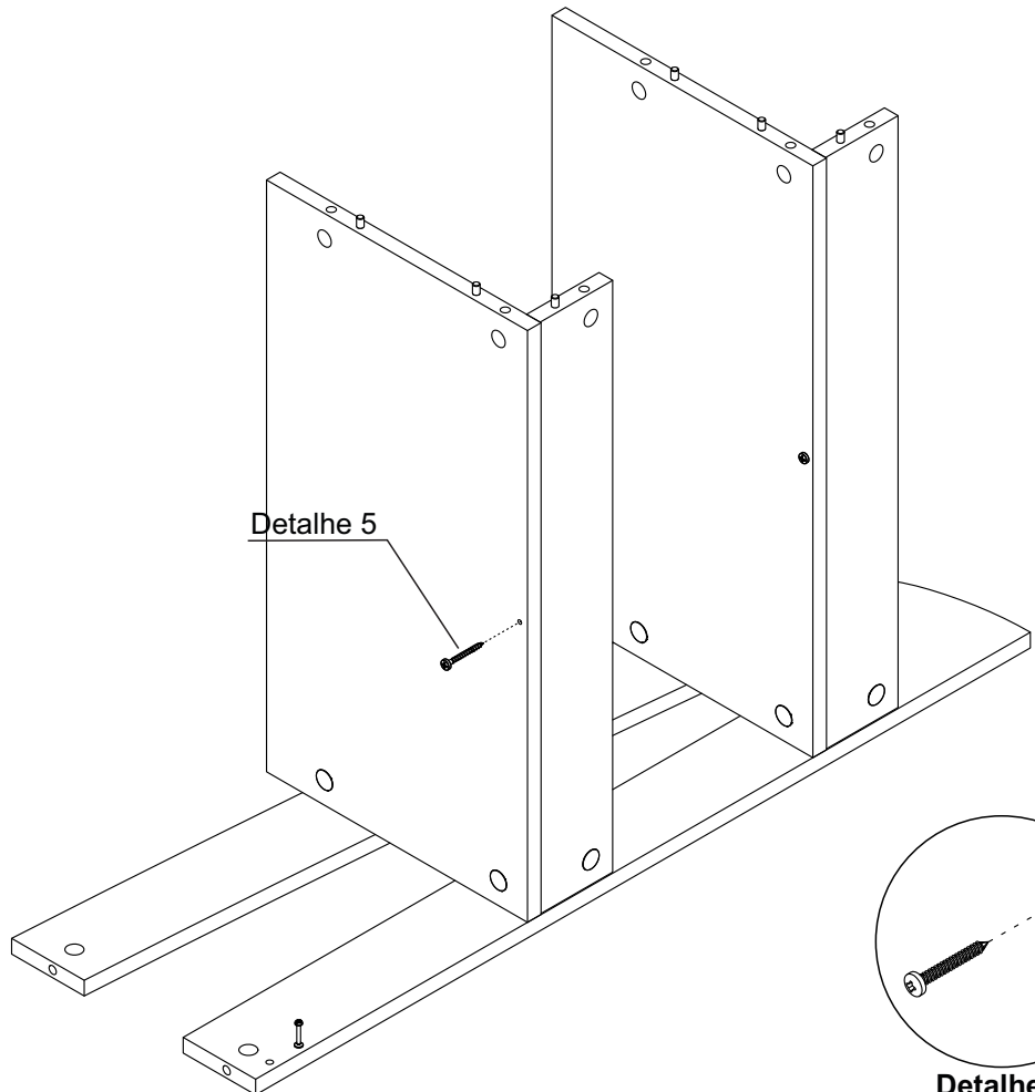
Detalhe 5 Detail/Detalle
