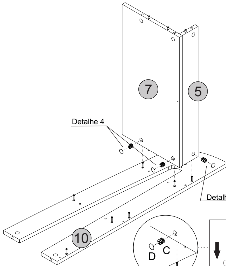
Detalhe 4 Detail/Detalle
