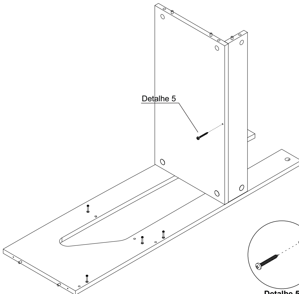
Detalhe 5 Detail/Detalle
