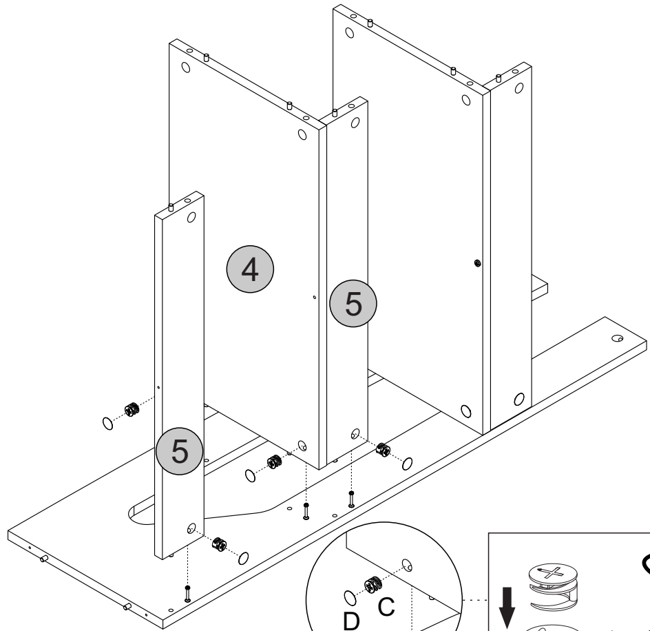
Detalhe 4 Detail/Detalle
