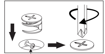
Detalhe 4 Detail/Detalle
