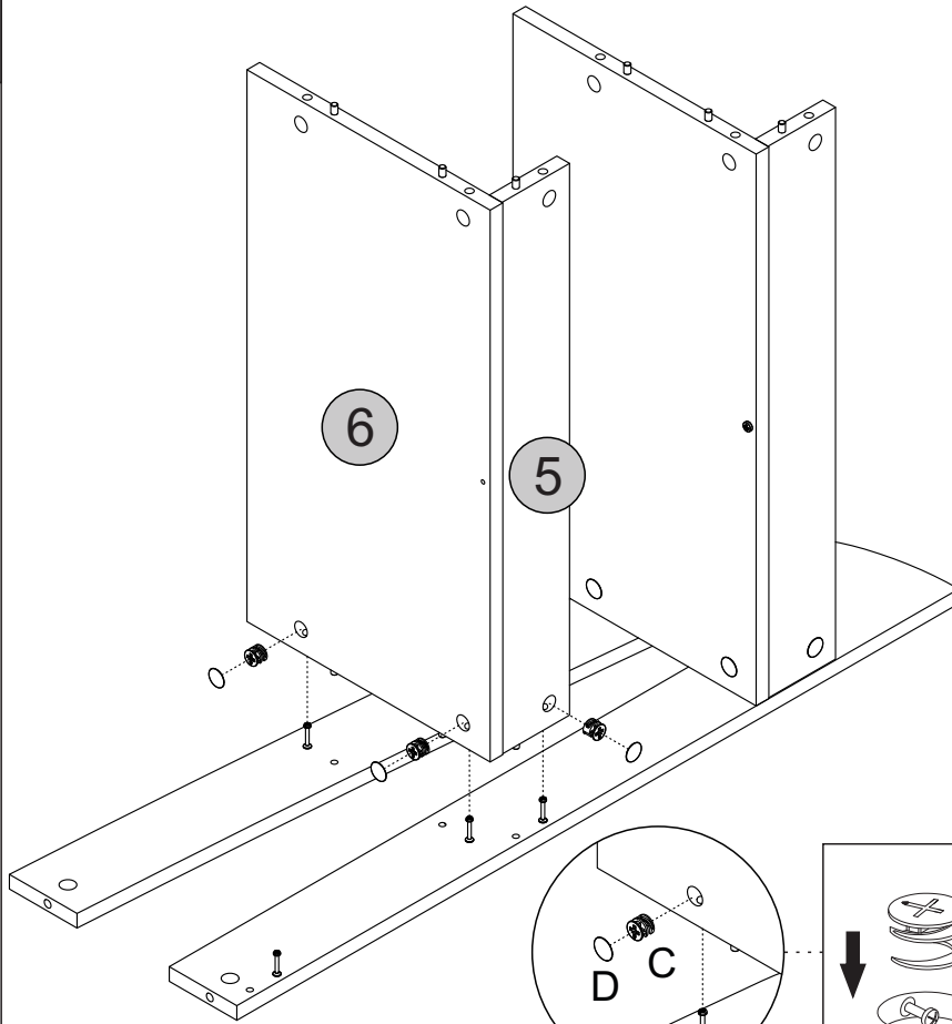
Detalhe 4 Detail/Detalle
