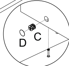
Detalhe 4 Detail/Detalle
