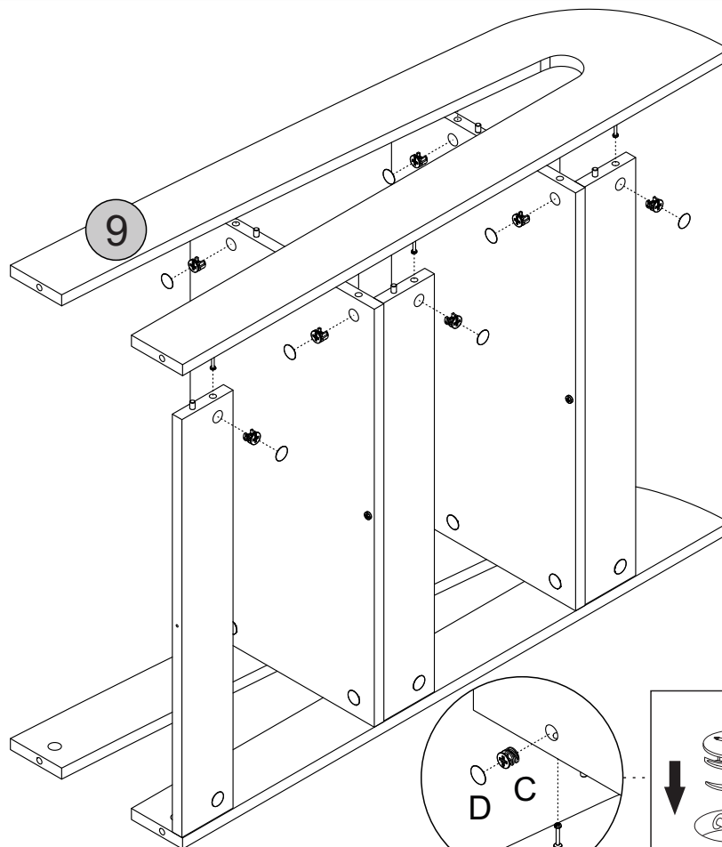
Detalhe 4 Detail/Detalle
