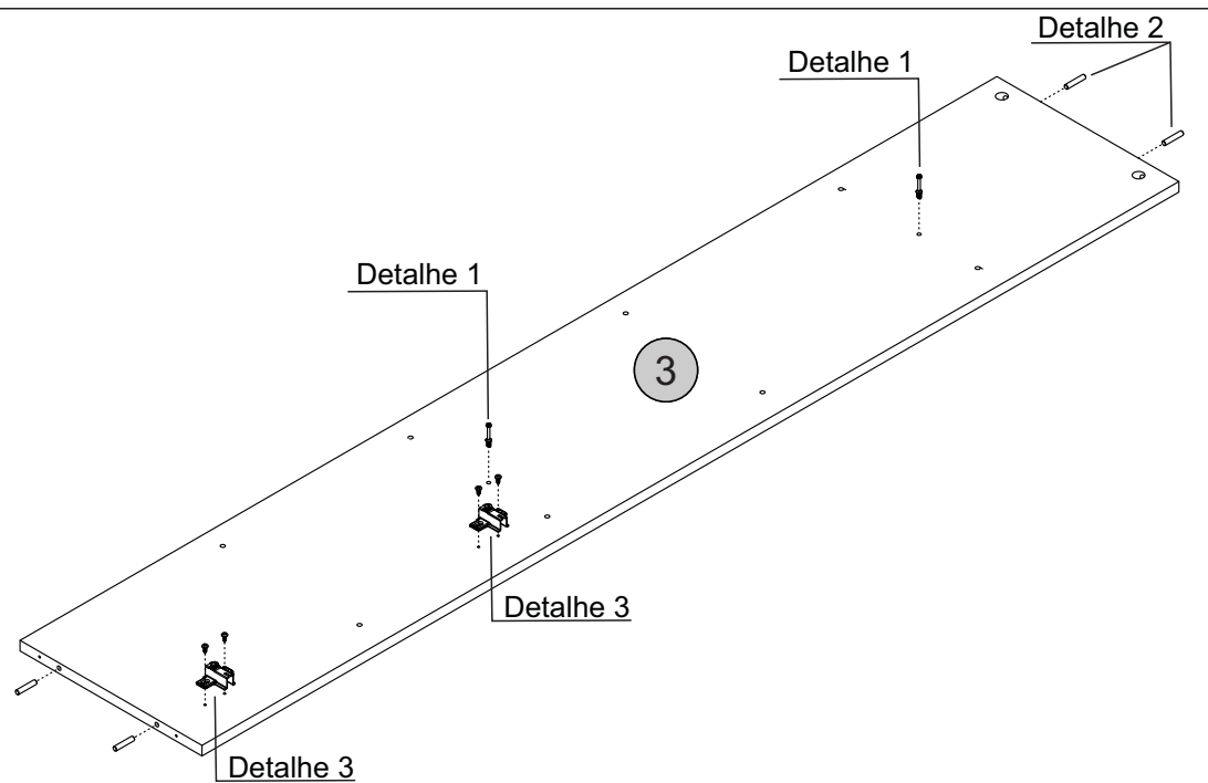
Detalhe 1 Detail/Detalle
